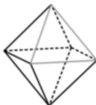
Ottaedro
