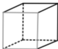
Esaedro
