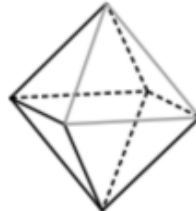
Ottaedro {3,4}
