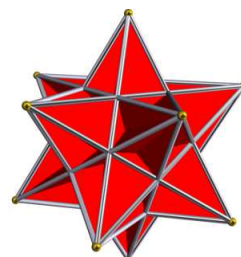
Grande icosaedro
