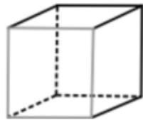
Esaedro {4, 3}
