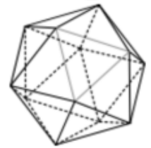
Icosaedro {5, 3}
